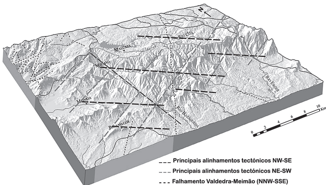
Figura 5 Rede de fraturação entre a Serra da Malcata e a superfície de Castelo Branco
