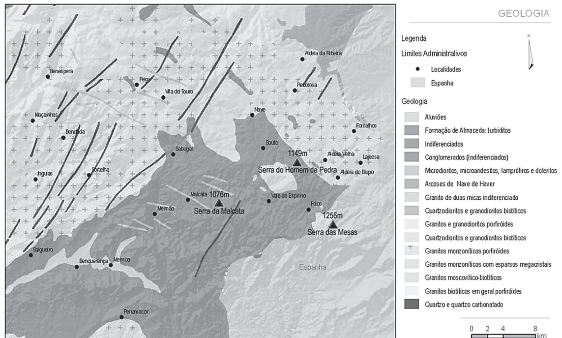
Figura 2 Mapa geológico da área de estudo
