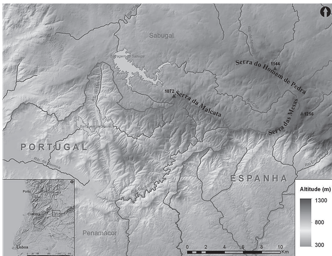
Figura 1 Mapa de enquadramento da Serra da Malcata
