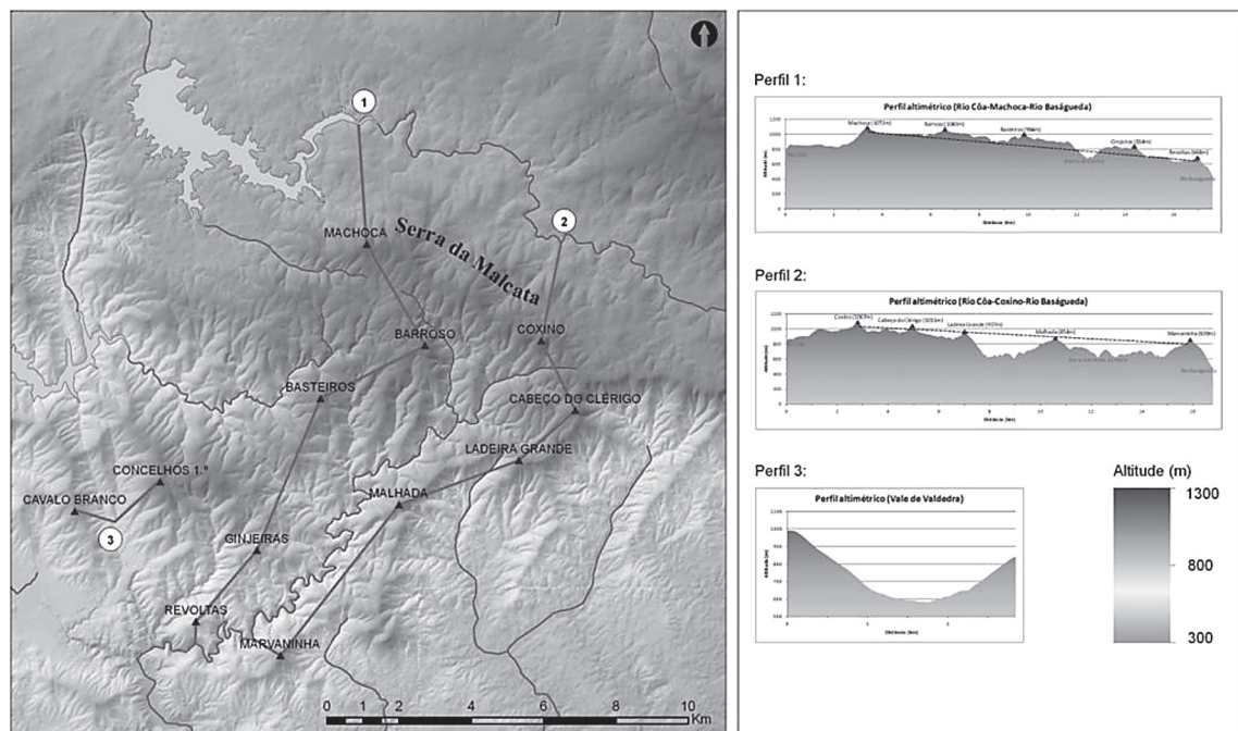
Figura 4 Perfis altimétricos da Serra da Malcata
