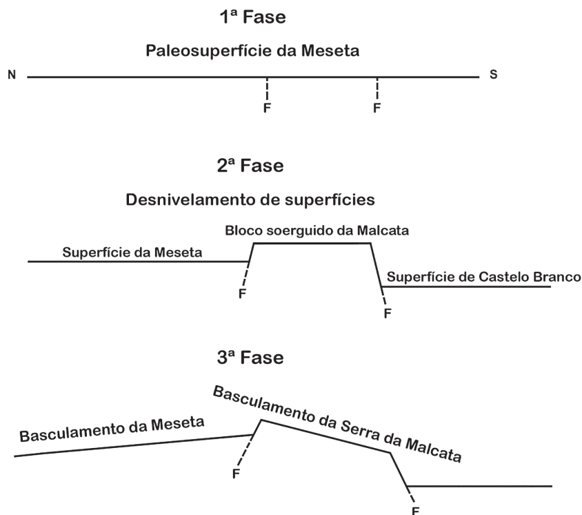
Figura 3 Esquema da evolução da Serra da Malcata
