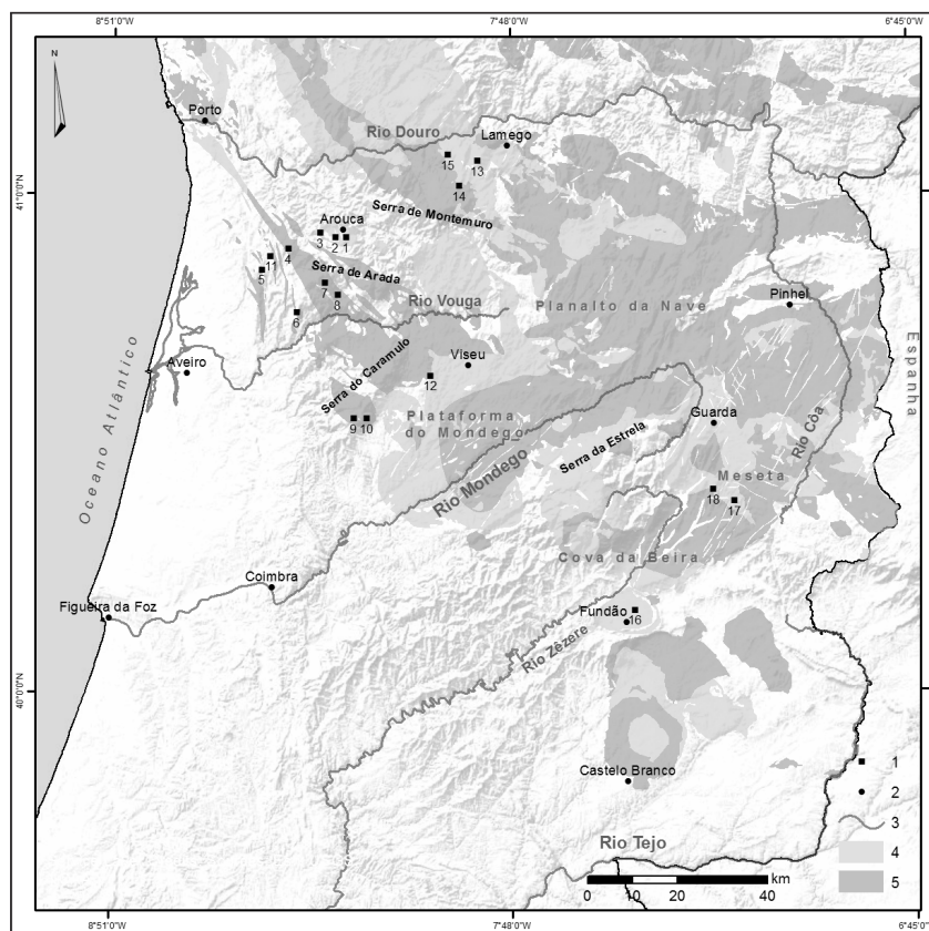
Figura 3 Localização das principais formas alveolares e a sua relação com as rochas graníticas do Portugal Central (adap. CORDEIRO, 2004: 2014).
