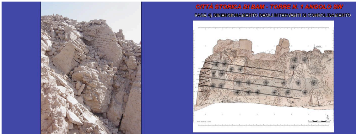
Fig. 5. Vista del estado del daño en la torre y plan de perforaciones ortogonales e inclinadas, para refuerzos de fibra de vidrio. Ciudadela de Bam, Irán. (Crédito: Ing. Valter Santoro, 2008).
