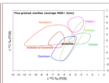
Figura 2- A: Cubierta de Sarcófago de Carranque (Toledo). B: Muestra. C: Lámina delgada. D: catodoluminiscencia. E: valores isotópicos de los principales mármoles blancos de grano fino (media MGS <2mm) (según Gorgoni et alii , 2002, Lapuente et alii , 2000, Attanasio et alii , 2015) con indicación de la localización de la muestra.
