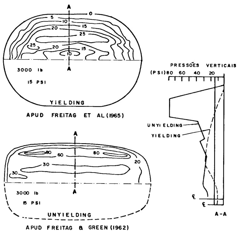
Fig. 6 — Pressão transmitida em função do aumento do grau de compactação.
