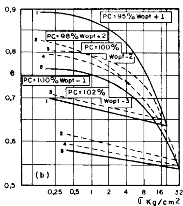
Fig. 2 — Compactação implica em pressão de preadensamento, não afectando perceptivelmente C_c (Índice de Compressão).
