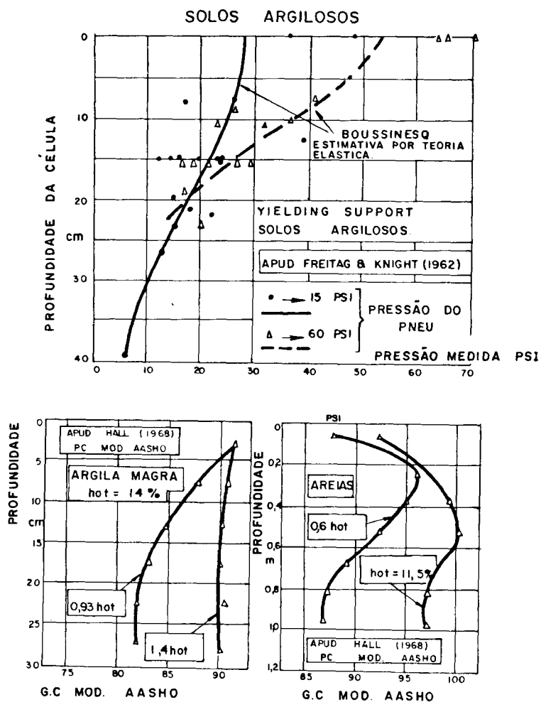
Fig. 5 — Distribuição de pressões em profundidade devido à compactação pneumática.
