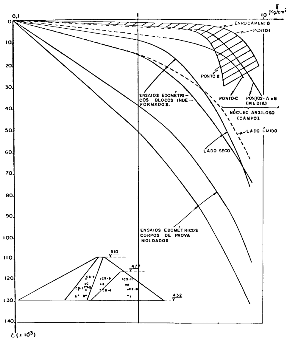
Fig. 19 — Dados de compressibilidade, laboratório e campo—Salto Santiago.
