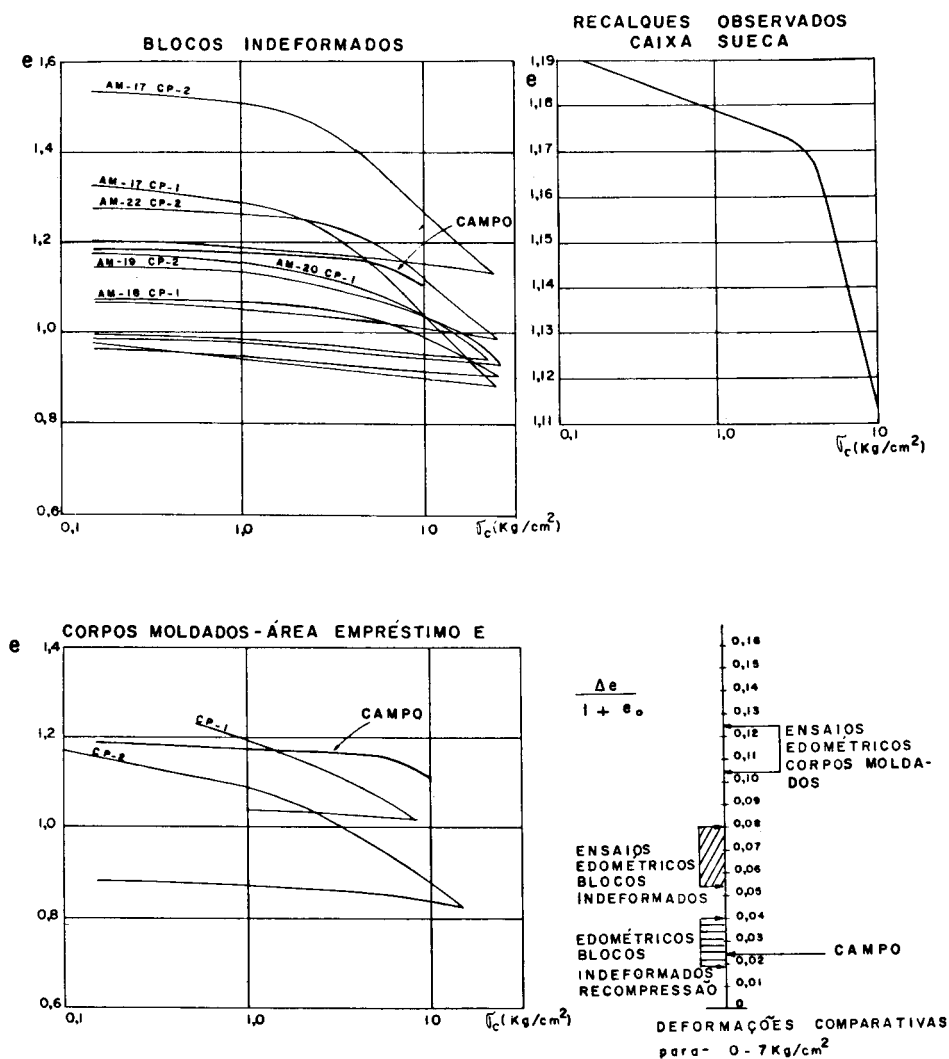
Fig. 18 — Dados de compressibilidade, laboratório e campo—Salto Santiago.
