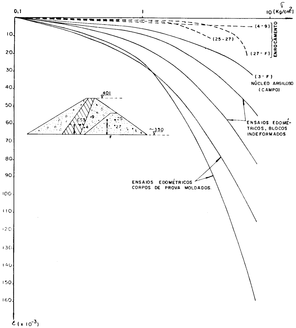
Fig. 17 — Dados de compressibilidade, laboratório e campo.
