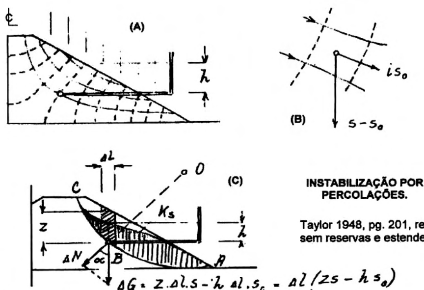
Fig. 2 – Indicação esquemática fundamental da postulação de Terzaghi (1936).
