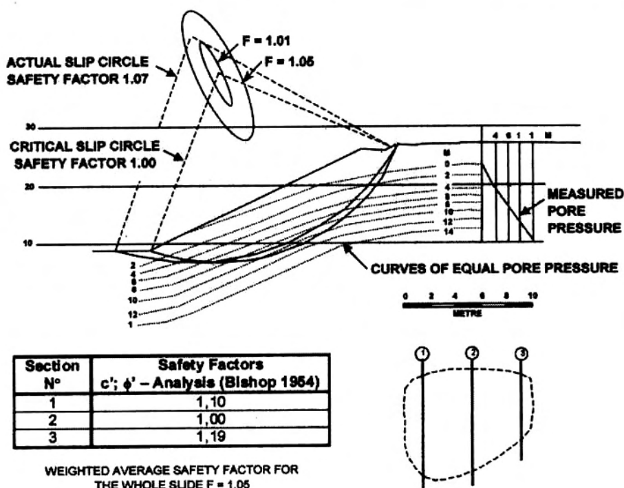
Fig. 5 – Dados de apoio a rupturas em F \equiv 1,00 (tensões efetivas e redução da resistência).
