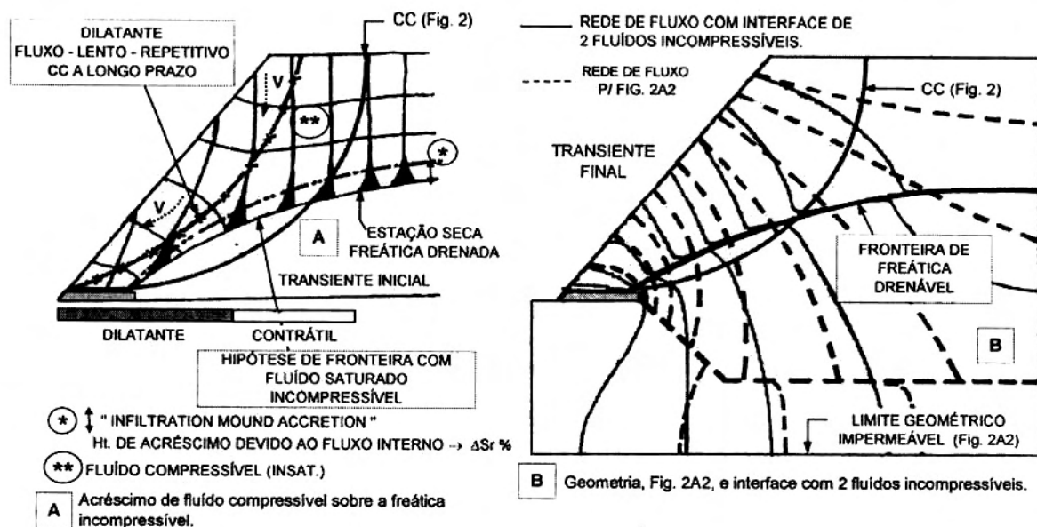
Fig. 8 – Instabilizações de taludes por redes transientes cabíveis de infiltrações pluviais sob análises mais amplas.
