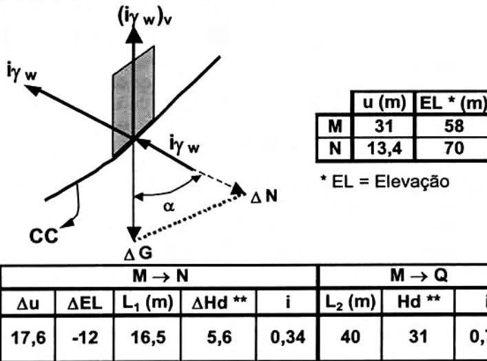
DETALHE 2 - Estática das Lamelas
