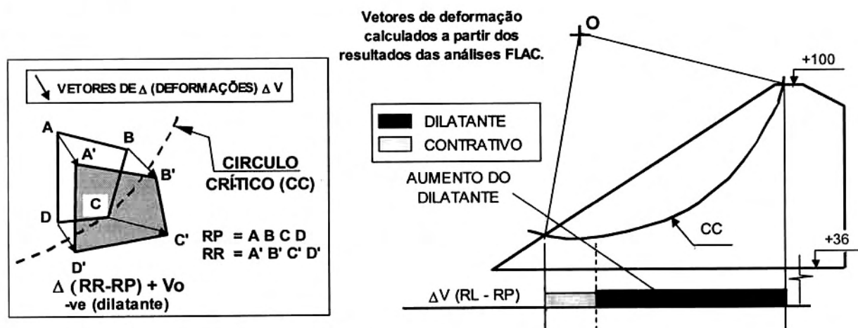
Fig. 7A – Redes, Vetores, Fs para RP e deslizamento raso sob RL ou RR.
