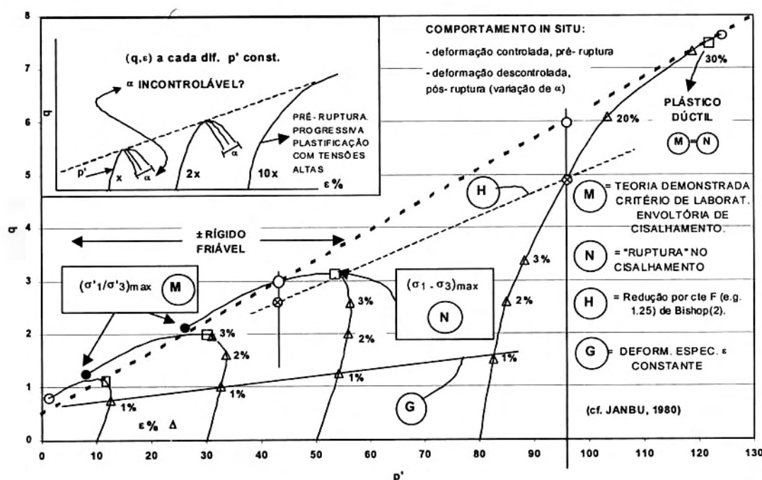
Fig. 10 – Apreciações básicas da geotecnia reconhecida ref. tensão-deformação, e resistências.
