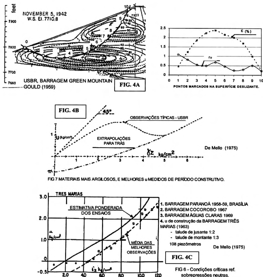
Fig. 4 – Pressões de FIM DE CONSTRUÇÃO FDC vistas sob fatores regionais diferentes.
