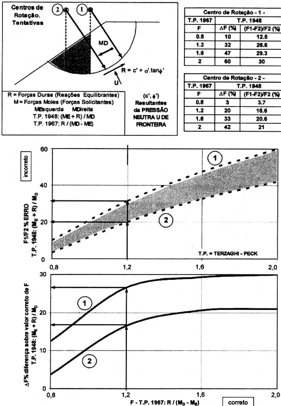
Fig. 3 – Erro conceitual, e não desprezível numericamente, pela “mistura” de cargas moles e duras.
