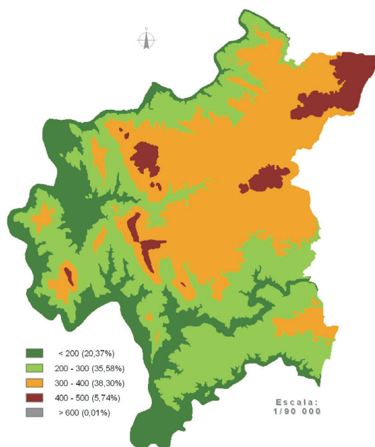
Fig. 1 - Mapa de classes altimétricas.
